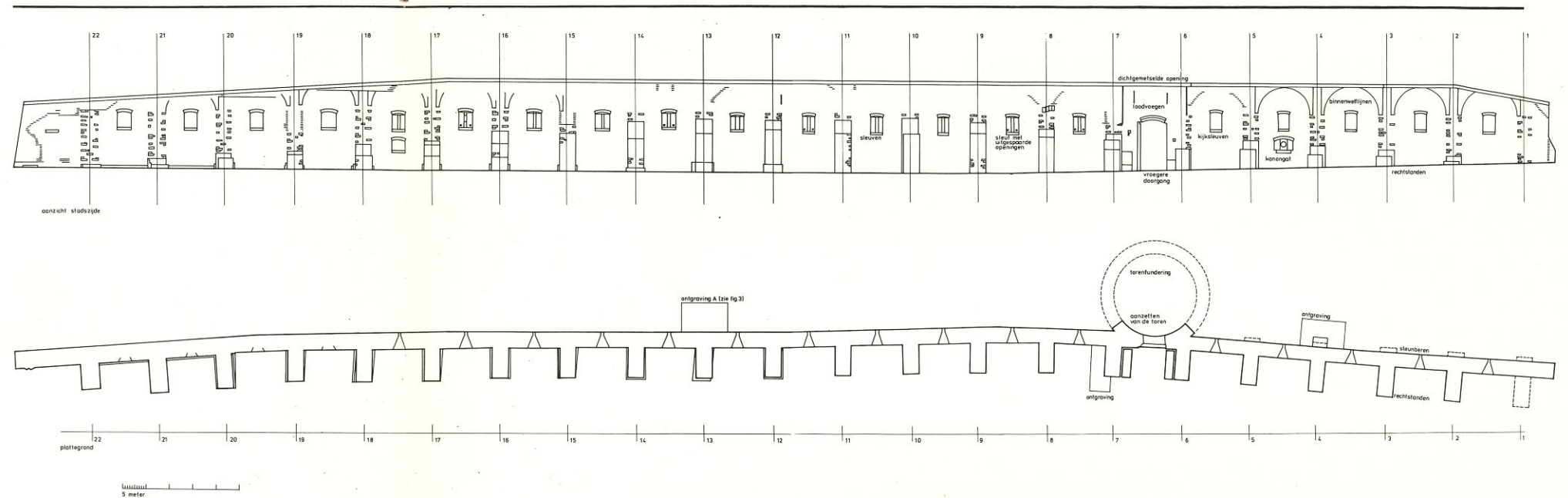
Figuur 2. Opmeting aan de stadszijde.
