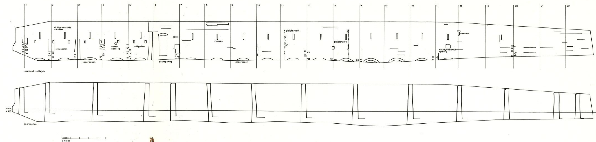
Figuur 1. Opmeting aan de veldzijde.
