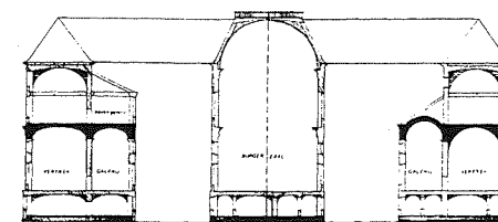
Doorsnede van het stadhuis van Amsterdam. Links het oorspronkelijke ontwerp van Van Campen, rechts de uitvoering onder leiding van Stalpaert.
