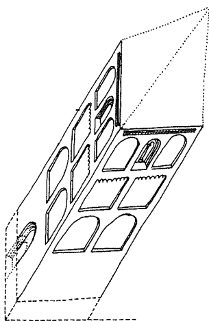
2. De toren van de Sint-Joriskerk. Reconstructie van de toestand rond 1200.
