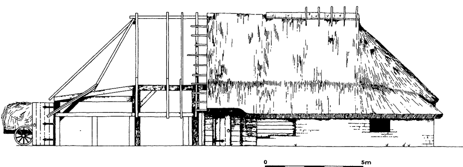
2. Deels lengte-doorsnede door, deels zij-aanzicht van de boerderij.
