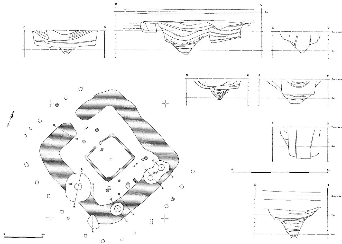
4. Links: plattegrond van de Romeinse greppelstructuur. Boven en rechts: verticale doorsnedes A-B t/m G-H.
