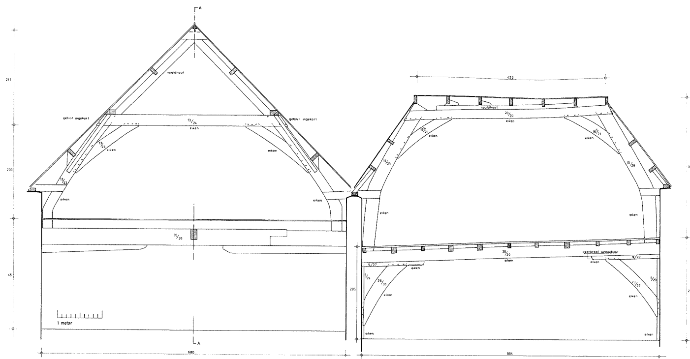
Doorsnede van tweede verdieping Langestraat 42 en 44. Tekening P. de Boer, Gemeentewerken Amersfoort.
